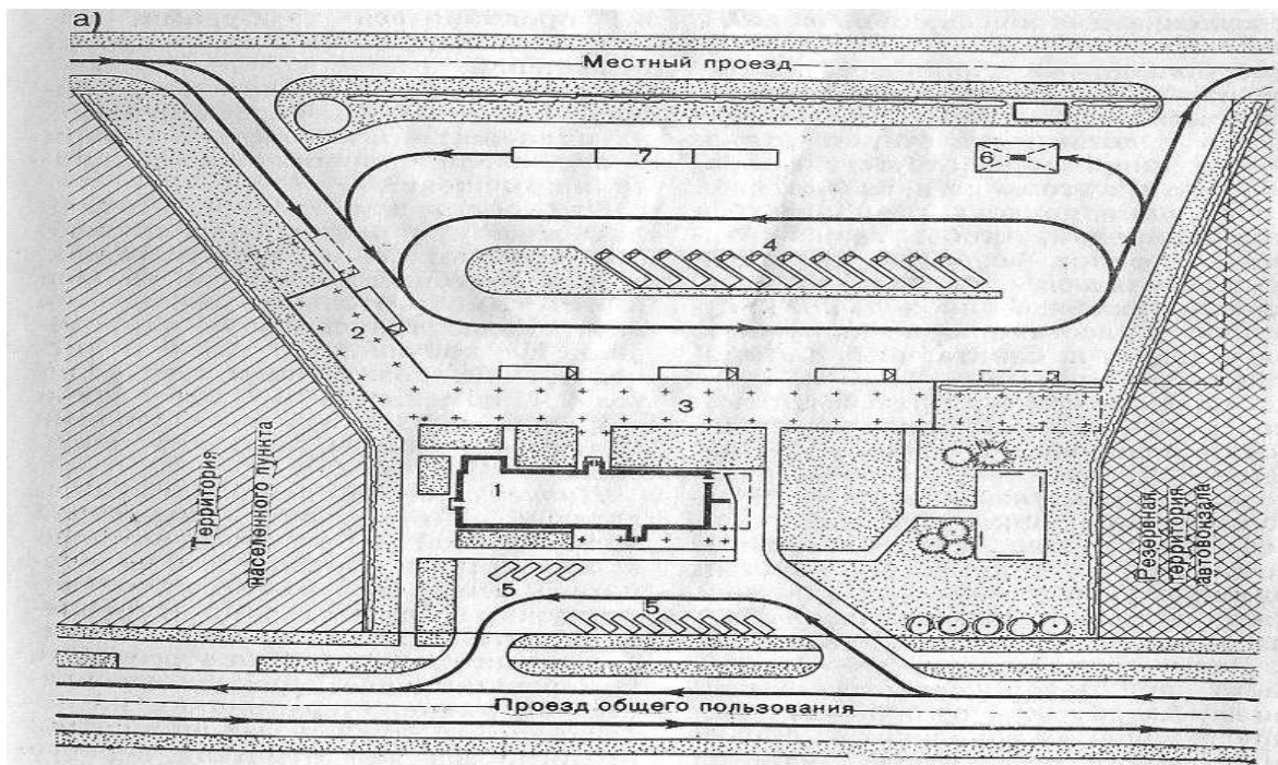
Рис. 28. Автовокзал вместимостью 100 чел. (типовой проект, Ленинградский филиал а — генеральный план; б — план 1 — пассажирское здание; 2 — перрон прибытия; 3 — перрон отправления; 4 — стоянка автобусов между рейсами; 5 — пассажирский зал; 6 — кассы; 7 — помещение для пассажиров с детьми; 8 — администрация; 9 — камера хранения багажа; 10 — торговый зал кафе; 11 — подсобные помещения; 12 — техническое помещение
