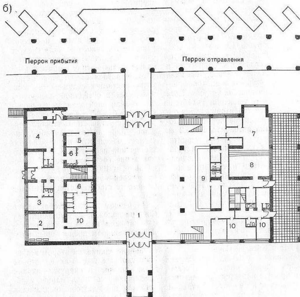
Рис. 32. Автовокзал в Суздале (Ленинградский филиал Гипроавтотранса, 1970 г., авторы С. Ф. Энтелис, Л. Н. Травина, С. М. Белый, Ю. А. Гольденберг, Э. Ю. Джигурда): а — общий вид; б — план первого этажа; в — план второго этажа:
