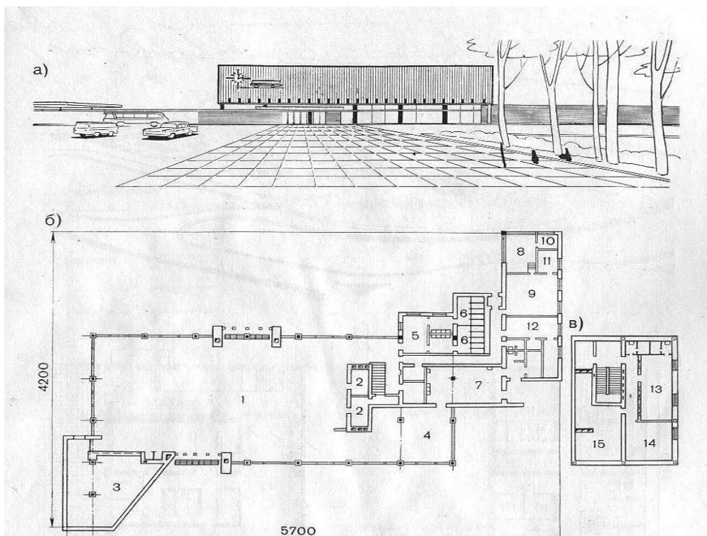
Рис. 31. Автовокзал в Калининграде (Ленинградский филиал Гипроавтотранса, 1967 г. авторы Л. М. Гольдвассер, В. В. Федорович, Э. С. Журавлева, Ю. А. Гольденберг, Э. Ю. Джигурда):
